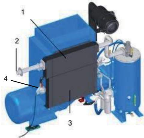
Рис. 11: Охладитель
