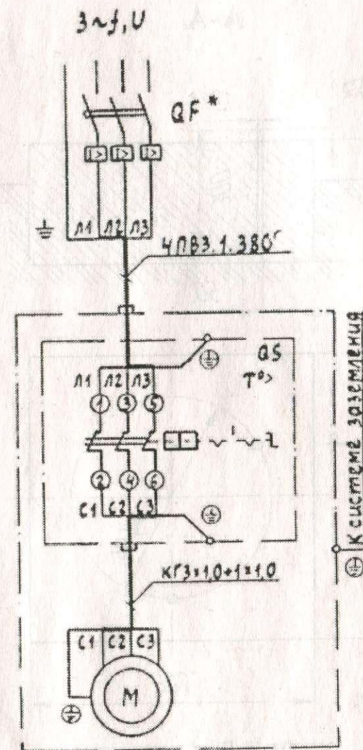
Рис. 12. Схема электрическая принципиальная и соединений установки компрессорной, модель KB-7
