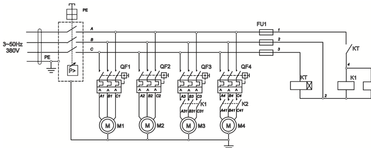
Рисунок А.2 - Схема электрическая принципиальная компрессоров СБ4-150.OLD20×4 и СБ4-150.OLD20×4/10
