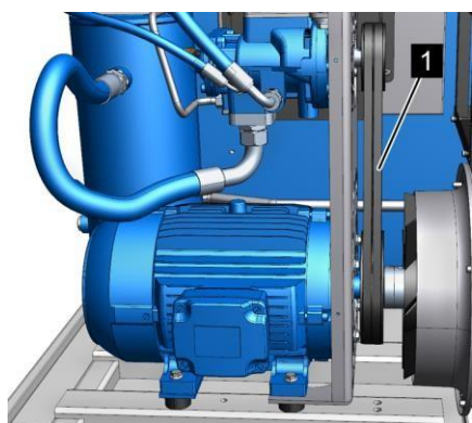
Рис. 15: Приводной агрегат
