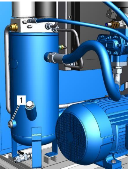
Рис. 30: Смотровое отверстие
